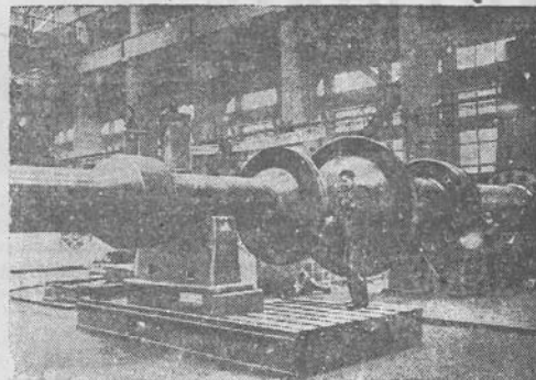
LENINGRADAS. Staline vardo fabrike hidroturbinų ceche. Vėjų paruošimas elinei Dniepro turbinai.
