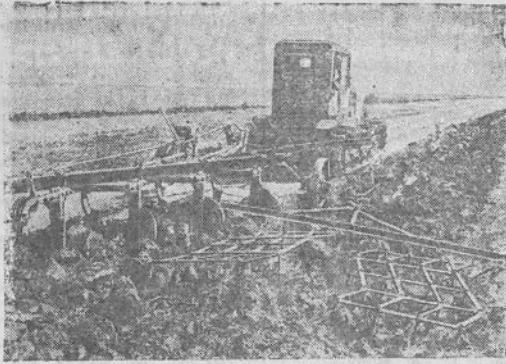
STAVROPOLIO KRAŠTAS. Drauge su pavasario sėja Petrovskio grūdų tarybiniam ūkyje vyksta ankstyvoji pūdyimo arimas. Traktorininkas N. Dymko kasdien traktorium „STZ — Nati“ pakelia po 7—8 ha pūdyimo, esant normai 5 ha. Nuotraukoje: traktorininko N. Dymko agregatas arime. Foto G. Arakeljano TASS'o spaudoje klisė.
