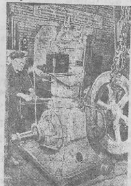
KAZANĖ. ISRS Žemės Ūkio Ministerijos mechaninis fabrikas įsivaivino didelių išleidimų 45 arklio jėgų galinamu, kurie bus skiriami mašinų — traktorių stotims bei kolektyviniams ūkiams. Nuotraukoje: Šalikavlis S. Sibgatullinas prie dizelio sustatymo. Foto B. Misanikovo TASS'o spaudos klisė.
