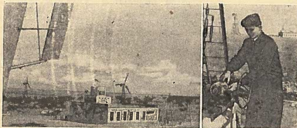
KAZACHIJOS TSR. Neseniai Akmolinsko srityje, netoli „Avangardo“ remonto-technikos stoties buvo atiduota eksploatuoti 400 kilovatų galingumo vėjinė elektros stotis.
