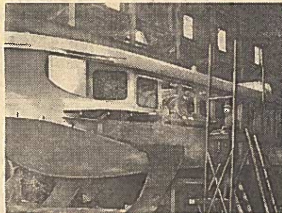
Gorkis. „Krasnoje Sormovo“ gamykloje statomas upinis šiluminis laivas su povandeniniais sparnais. Laive tilps 66 keleiviai. Laivas galės išvystyti greitį iki 60 km per valandą.
