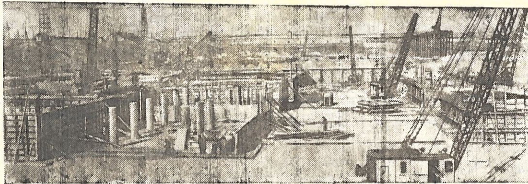
KACHOVKOS HIDROMAZGO STATYBOJE. Laivybos šliuzo statyboje prasidėjo armatūros įrengimas ir šliuzo antrosios eilės betonavimas. Sparčiai auga HES pastatas ir vandens užtvanka. Nuotraukoje: bendras hidroelektrinės ir vandens užtvankos statybos vaizdas. J. Lichuto (TASS) nuotrauka.
