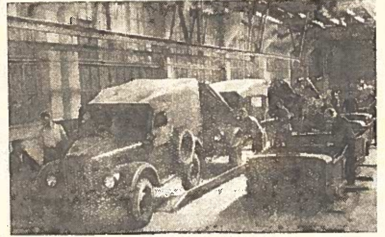
GORKIS. V. M. Molotovo vardo automobilių gamykloje sukurtas naujas automobilis „GAZ-69“. Naujoji masina puikiai nugalė smėlį, sniegą, pelkėtas vietas, kalnų perėjas. Jos didžiausias greitis — 90 kilometrų per valandą. Blogais keliais ji gali važiuoti 40–50 kilometrų greičiu. Aukštas mašinos eigumas, jos eiginiai savumai ir didelis ekonomiškas prisidės prie pačių nuošaliausių mūsų Tėvynės kampelių automobilizavimo. Nuotraukojė: automobilių „GAZ-69“ surinkimo ceche. V. Chramcovo (TASS) nuotrauka.
